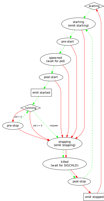
图 3 upstart 状态迁移
